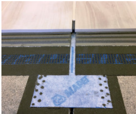
Mapeband Easy τοποθετημένο σε αρμό ελέγχου τουτσιμεντοκονιάματος
